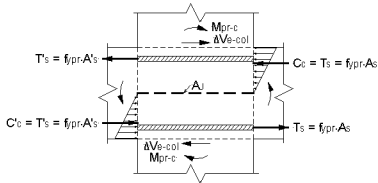
FIGURA 33 FUERZAS CORTANTES EN EL NUDO
