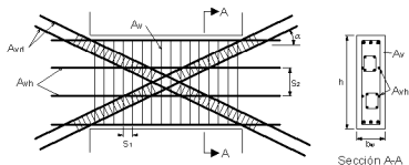
FIGURA 38 VIGA DE ACOPLAMIENTO
