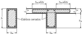
FIGURA 17 EL ÁREA SOMBREADA ES A_{OH}
