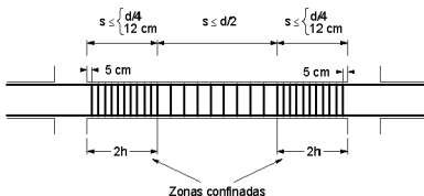
FIGURA 16 ZONAS CON REFUERZO DE CONFINAMIENTO
