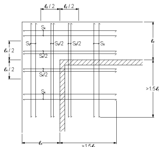
FIGURA 22 ARMADURAS EN VUELOS
