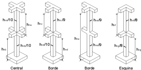
FIGURA 27 SOPORTE LATERAL DE LAS COLUMNAS
