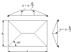
FIGURA 24 DISTRIBUCIÓN DE CARGAS SOBRE LOS APOYOS
