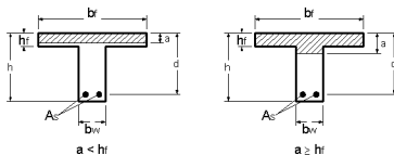
FIGURA 11 CASOS EN EL DISEÑO DE VIGAS "T"
