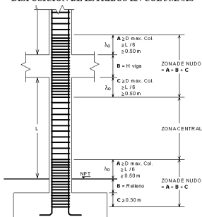
FIGURA 32 DISPOSICIÓN DE ESTRIBOS EN COLUMNAS
