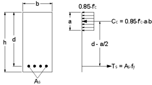
FIGURA 9 FUERZAS INTERIORES DE LA SECCIÓN
