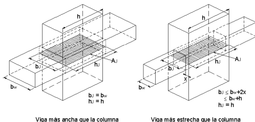
FIGURA 34 ÁREA EFECTIVA EN EL NUDO A_J
