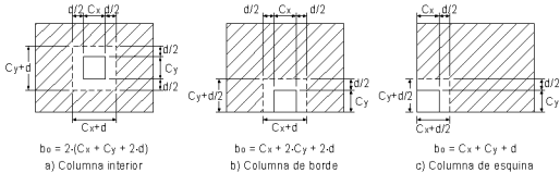
FIGURA 43 SECCIÓN CRÍTICA PARA CORTANTE COMO LOSA (PUNZONADO)
