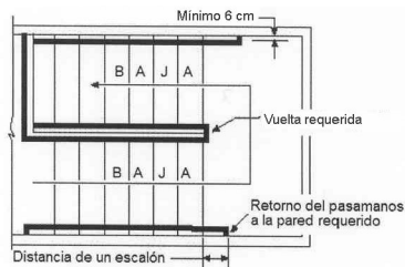
FIGURA 5 VISTA EN PLANTA DE LOS PASAMANOS.
