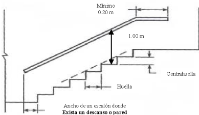
FIGURA 4 ALTURA DE LOS PASAMANOS
