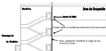
FIGURA 1 RECORRIDO DE UN MEDIO DE EGRESO
