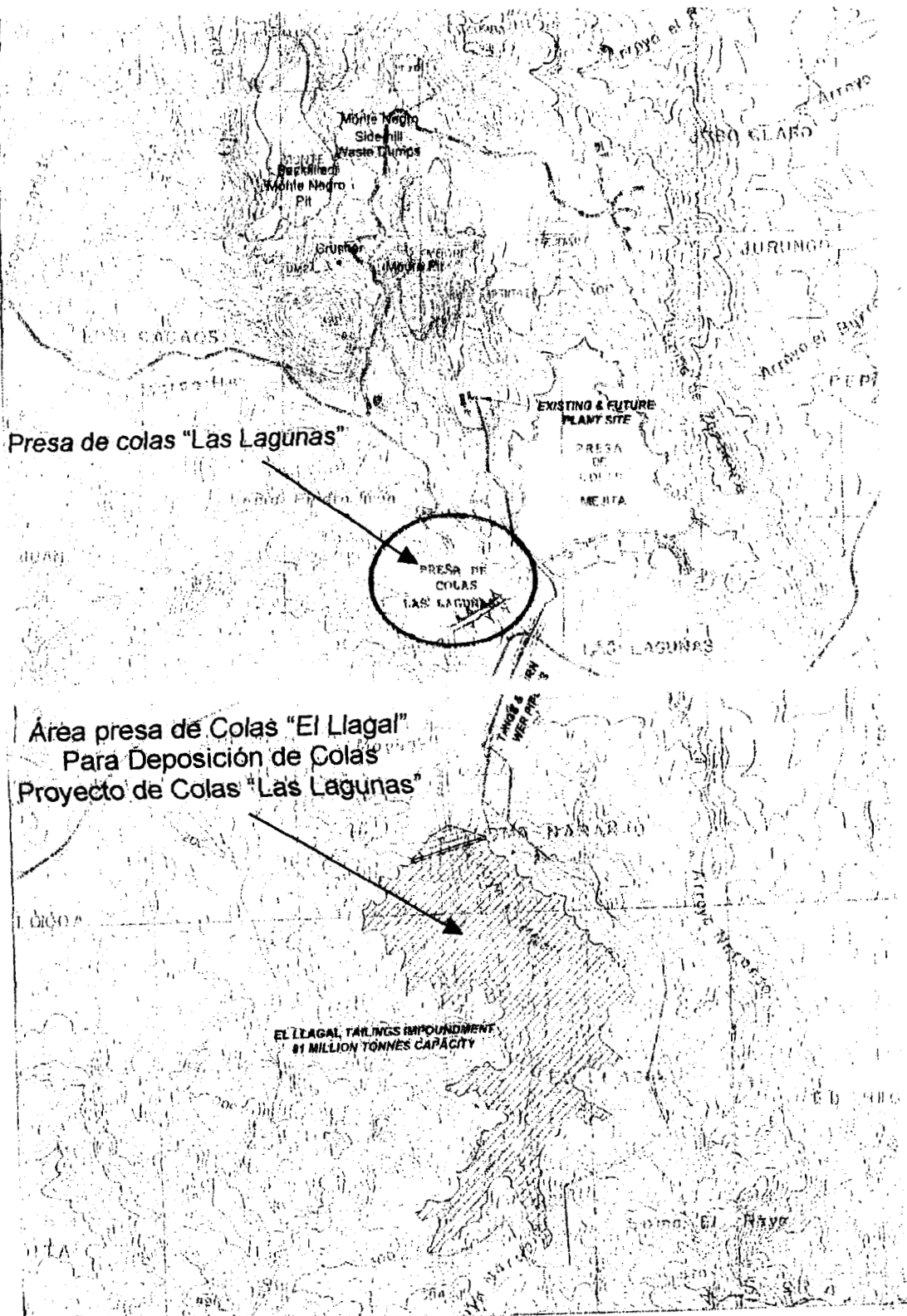
Anexo A, Figura No.4 Plano Mostrando el Area de la Presa "El Llagal"
